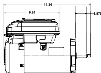
ECM16CU
